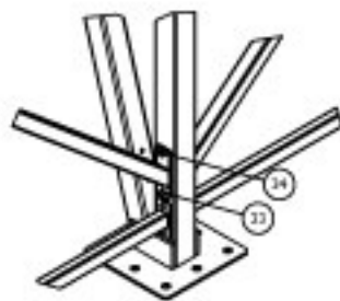
E (1:10)
